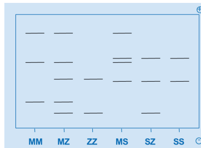
Abb. 3: Darstellung der \alpha_1 -Antitrypsin-Phänotypen durch isoelektrische Fokussierung (pH 4.2-4.9).
