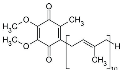
Abb. 1: Struktur von Coenzym Q10 (Ubichinon-10)
